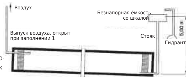
Рис. 10 Проверка герметичности
