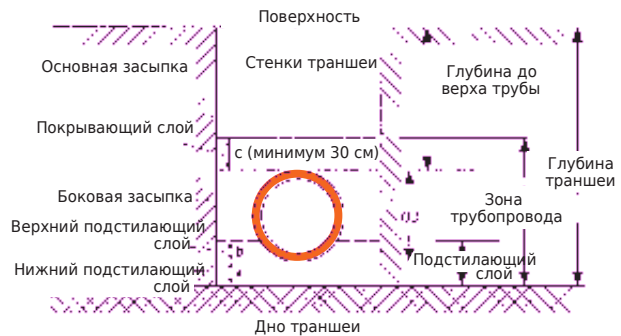
Рис. 3 Устройство траншеи
